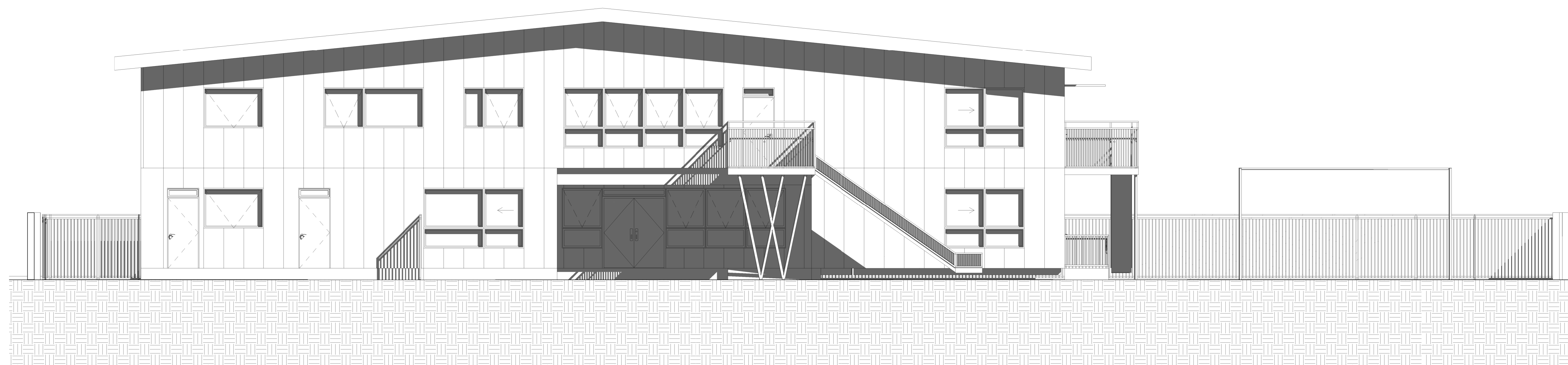
3 Elev Oriente 1 : 50
