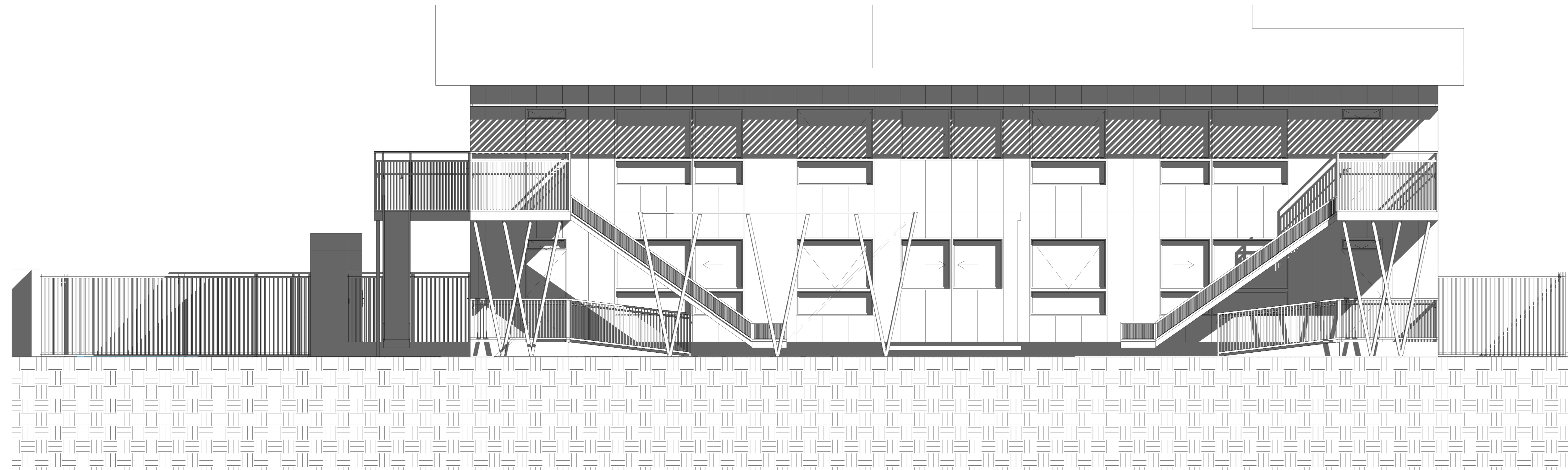
1 Elev Norte - Aulas 1 : 50
